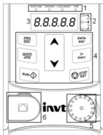
Figura 4-1 Consola tipo film
