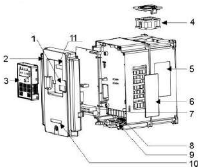
Figura 2-4 Estructura del producto (3Ø 400V \geq 4kW y 3Ø 230V \geq 1.5kW)
