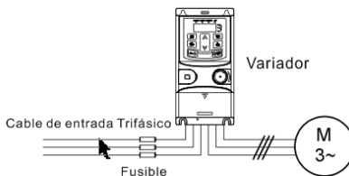
Figura 3-14 Configuración de la protección eléctrica
