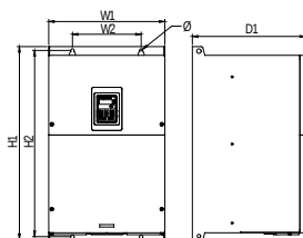
Montaje en fondo de armario de los variadores 3Ø400V 90~110kW (mm)
