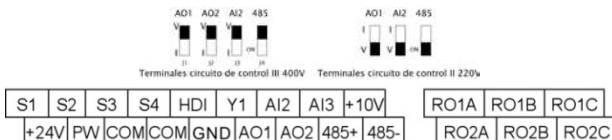
Figura 3-10 Terminales del circuito de control
