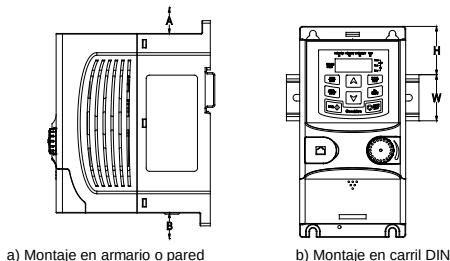
Figura 3-1 Instalación
