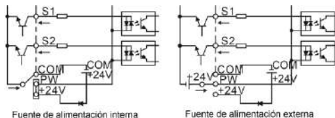
Figura 3-12 Modos de conexión NPN
