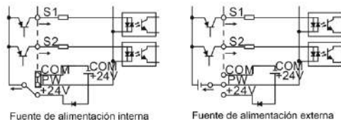
Figura 3-13 Modos de conexión PNP
