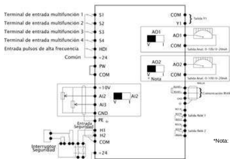
Figura 3-9 Diagrama de conexión del circuito de control Salida Relé 1
