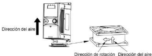
Instalación del ventilador en variadores 1Ø 230V / 3Ø 400V \leq 2.2\text{kW} y 3Ø 230V \leq 0.75\text{kW}
