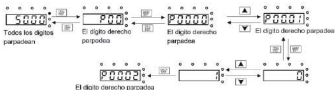
Figura 4-4 Gráfico esquemático de la modificación de parámetros
