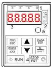
Figura 4-2 Consola extraíble
