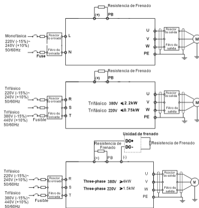
Figura 3-3 Diagrama de conexiones del circuito principal
