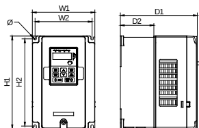
Montaje en fondo de armario de los variadores 3Ø400V ≥ 4kW y 3Ø230V ≥ 1.5kW (mm)
