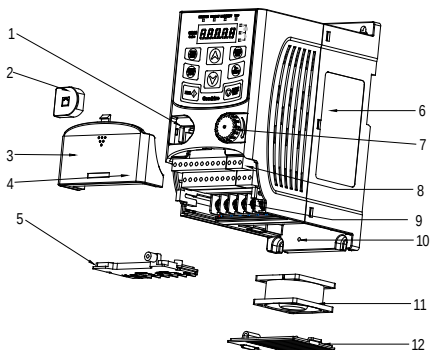
Figure 2-3 Diagrama del producto (1Ø 230V-3Ø 400V \leq 2.2kW y 3Ø 230V \leq 0.75kW)
