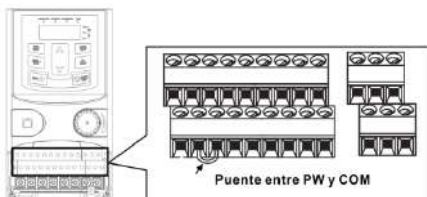
Figura 3-11 Puente entre COM y PW
