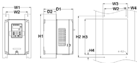
Montaje en brida (flange) de los variadores 3Ø400V≥4kW y 3Ø230V≥1.5kW (mm)
