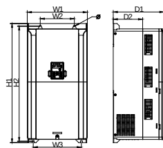
Montaje en fondo de armario de los variadores 3Ø400V 45~75kW (mm)
