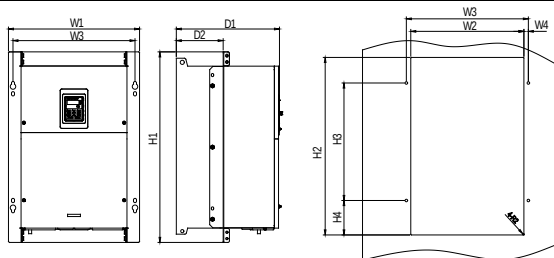
Montaje en brida (flange) de los variadores 3Ø400V 90~110kW (mm)
